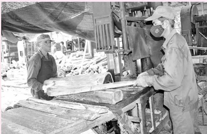
Sản xuất chế biến gỗ tại Công ty TNHH Công nghiệp Hòa Phát, huyện Yên Bình.
